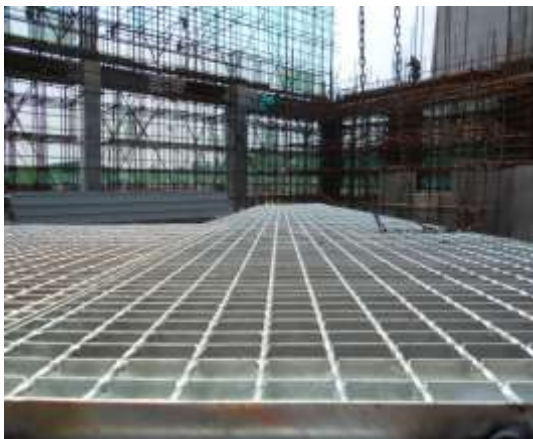
反應塔鋼平臺安裝
