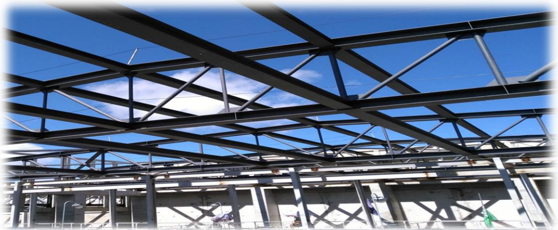
鋼屋架吊裝
