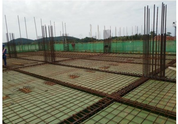
卸料平臺板底鋼筋綁紮
