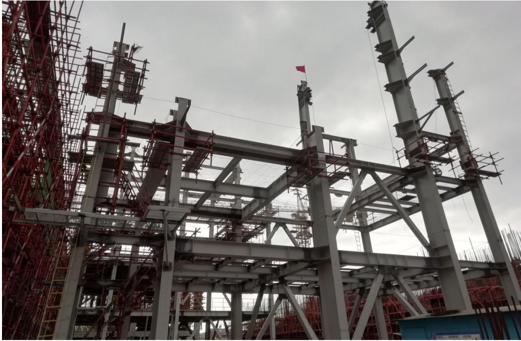
#2 焚燒爐鋼架吊裝
