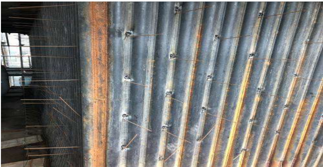
鍋爐本體保溫鉤釘外衣支撐焊接
