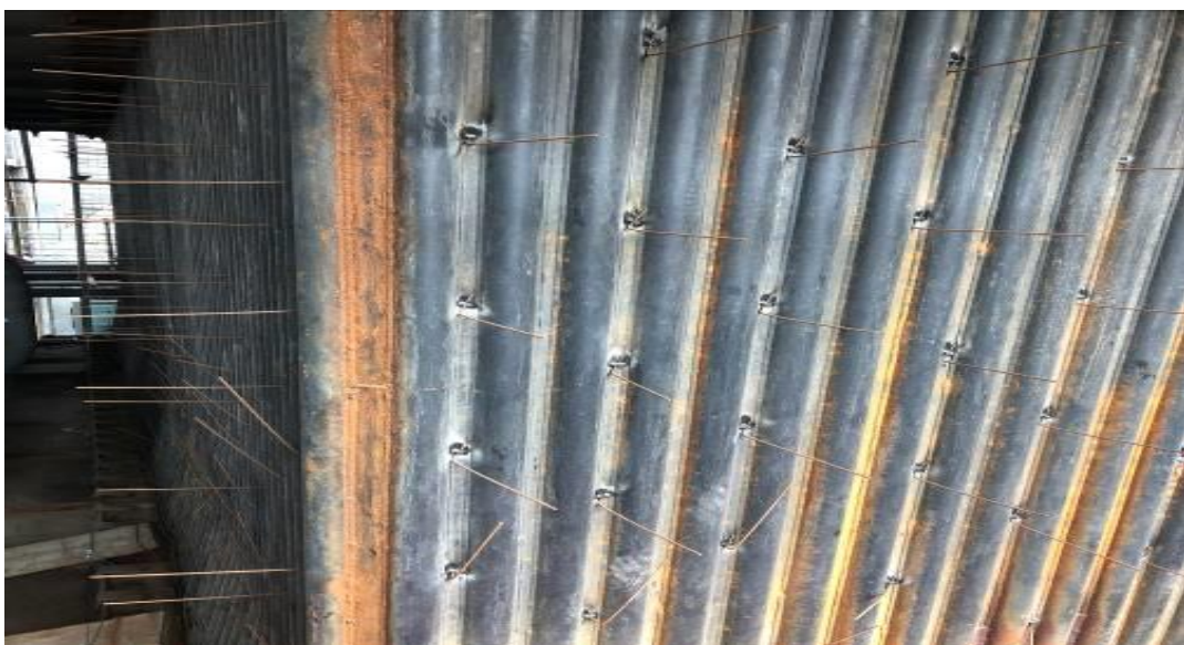
鍋爐本體保溫鉤釘外衣支撐焊接
